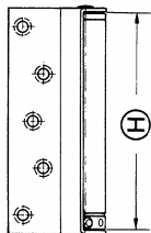
Charnière simple action Porte gauche Left-hand door
